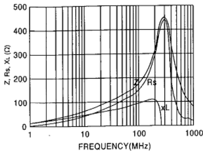
FI 63.5x15x12.7
