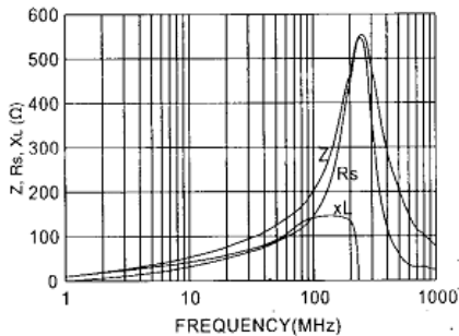
FI 63.5x15x12.7
